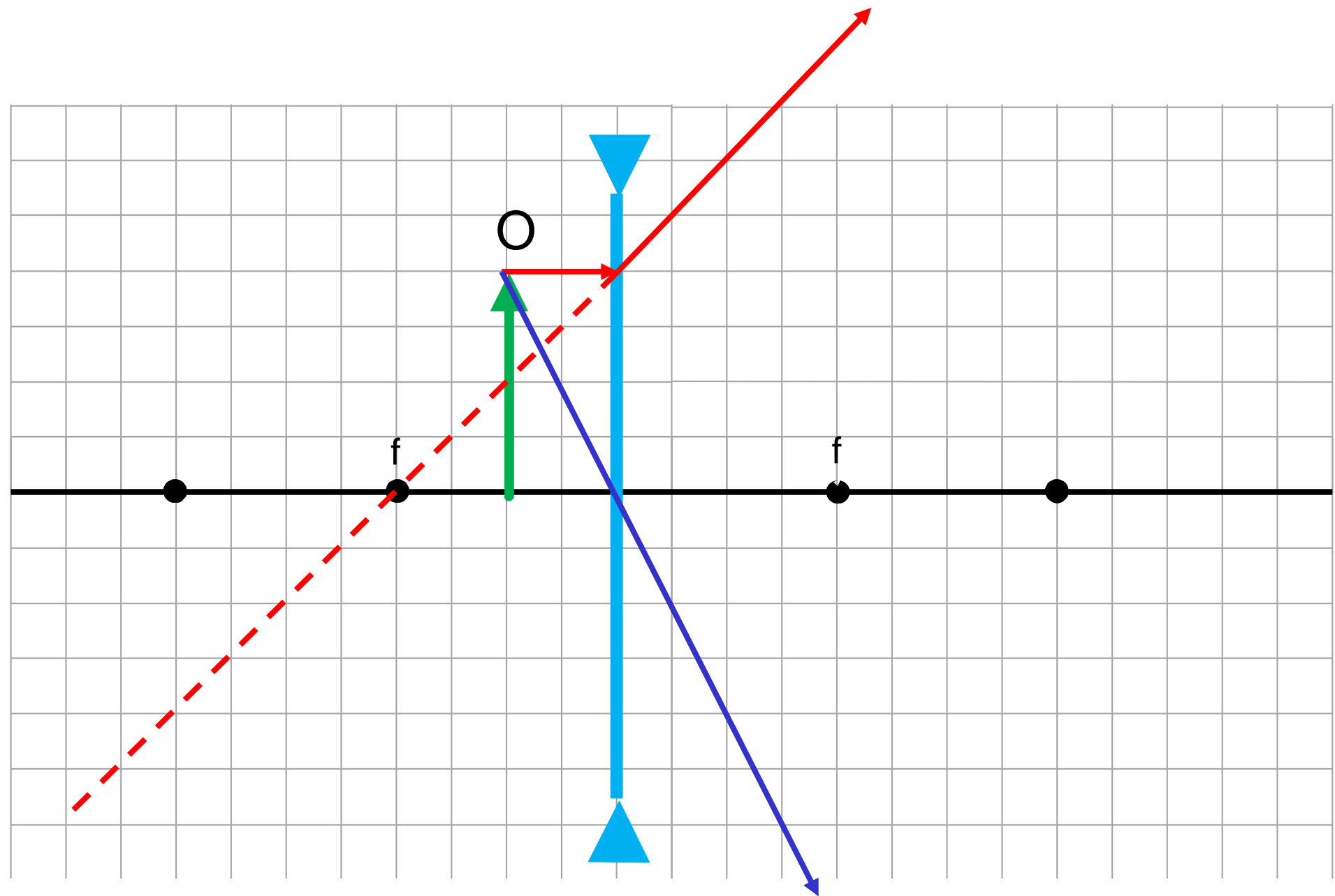
Figura 7: Objeto entre o vértice e o foco
