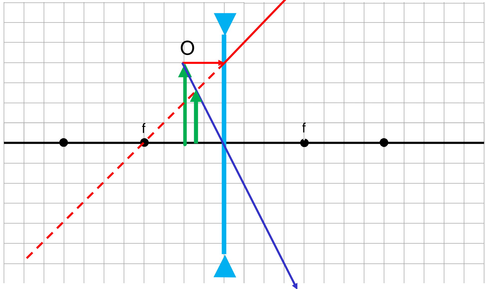
Figura 7: Objeto entre o vértice e o foco
