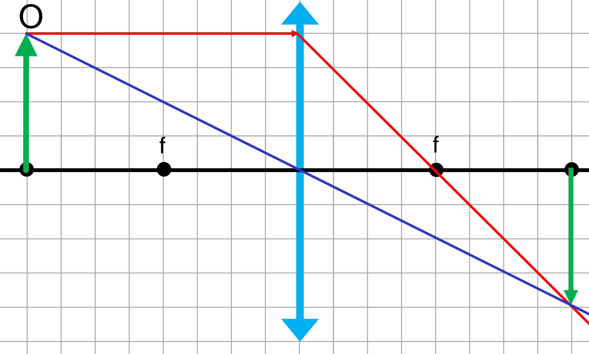
Figura 4: Objeto no anti-principal
