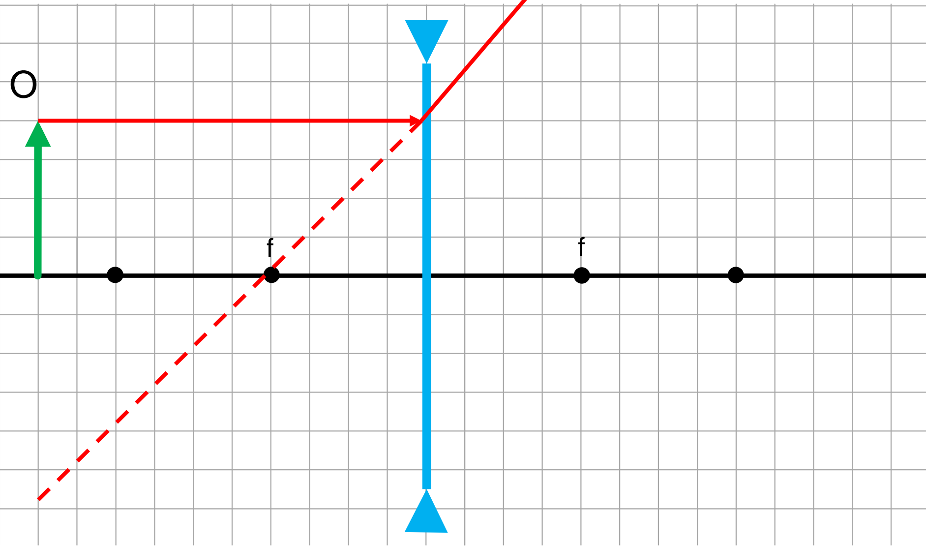
Figura 11: Objeto além do anti-principal
