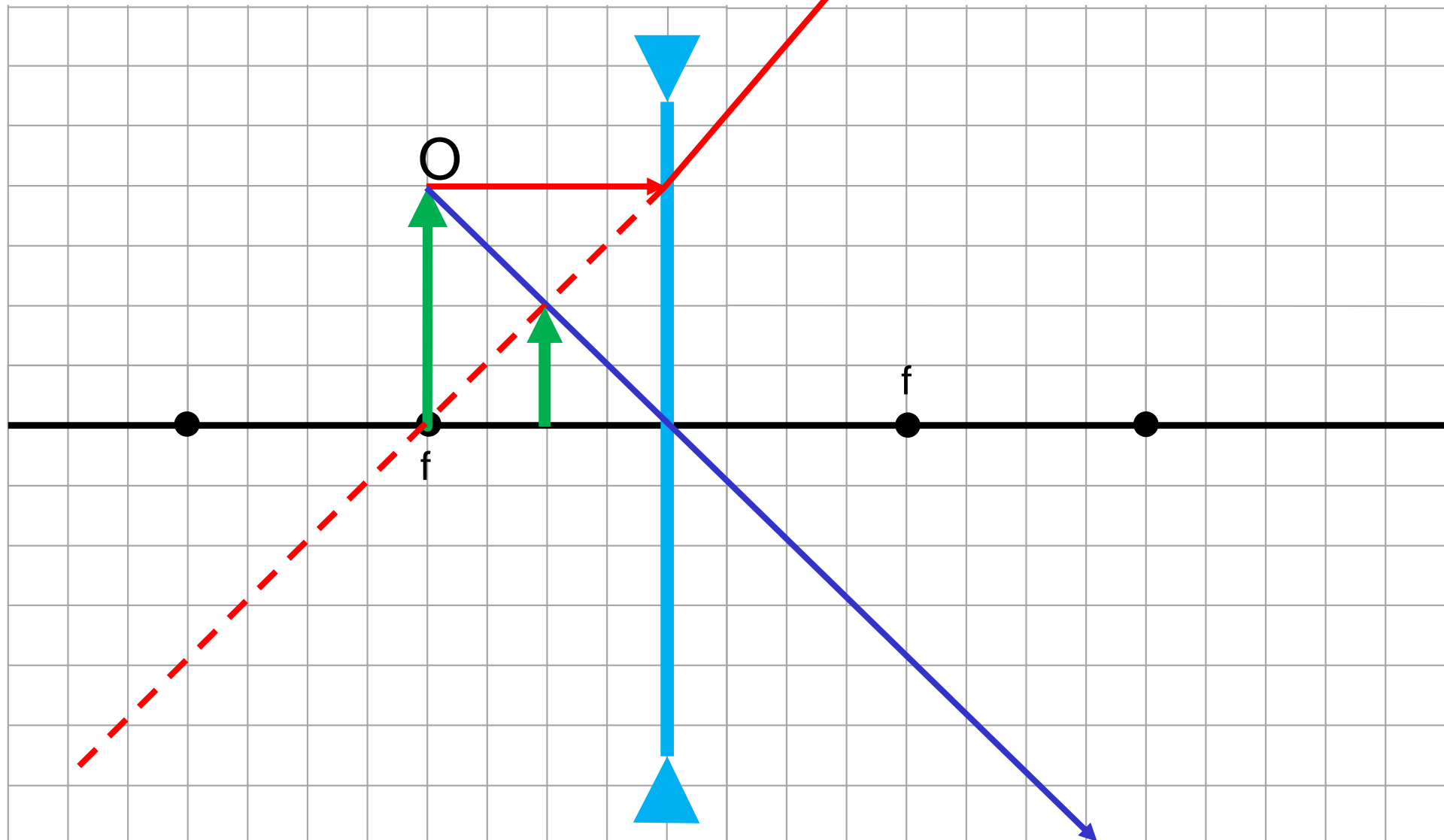
Figura 8: Objeto no foco
